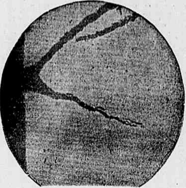
Os rompimentos das adutoras são ocasionados porque os canes que a Prefeitura emprega, fornecidos pela companhia americana Tetra, se corrompem facilmente. Na foto uma micrografia ampliada de um corte longitudinal em um arame do revestimento dos tubos da 4ª adutora, na altura do quilômetro 47, mostrando como está corroído
