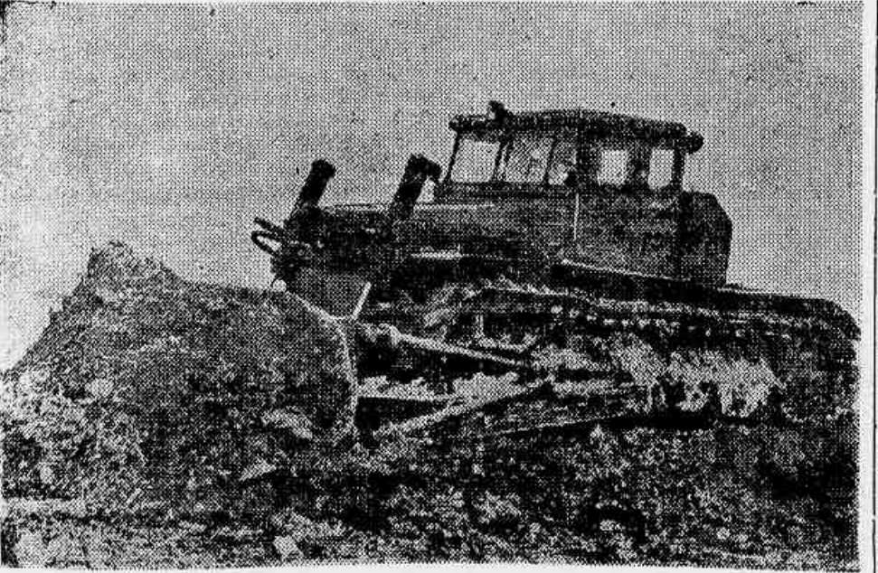
O trator Chelabinsk, produzido agora pelas fábricas soviéticas, é impulsionado por 250 cavalos vapor e dispõe de dirigibilidade elétrica. Sua cabina possui ar condicionado e permite uma ampla visibilidade ao tratorista. Na foto, o trator em funcionamento.
