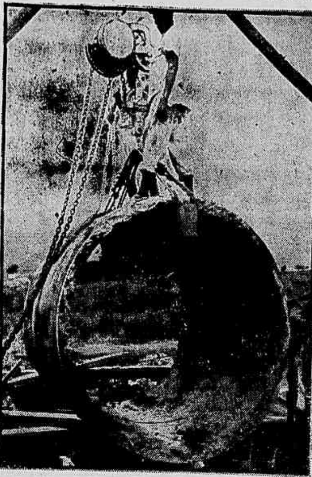
Apesar de todos os pareceres em contrário, inclusive de uma Comissão da Câmara dos Vereadores, foram usados para a terceira Adutora do Rio Guandu, os tubos da "Lock Joint", condenados por serem susceptíveis de uma corrosão violenta. (Stress Corrosion)
