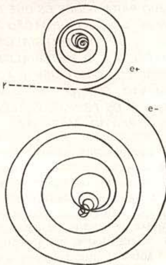
Fotografias tiradas numa Câmara de Bolhas apresentam este aspecto. Nesta vê-se que um raio de alta energia ( \gamma ) transformou sua massa e energia em um elétron e um pósitron, que giram em espirais devido ao campo magnético da câmara. O desenho realça a trajetória das partículas.
